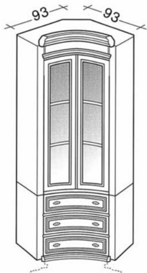
Art. 1510 Modulo Bizantino angolo 2 porte vetro Element 2 door corner piece Modul eckelement 2-türig 93x93x226 m3 0,94
