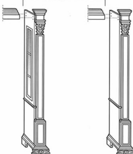
Art. 1532 Modulo Bizantino vetro gancio ponte dx-sx Element glass, hook, benches, dx-sx Modul Glas, Haken, Sitzbänke dx-sx 15x45x226 m3 0,15
